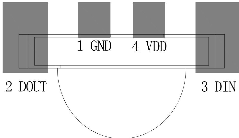
侧面贴装示意图
