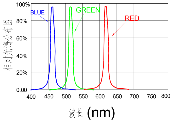
波长特性
