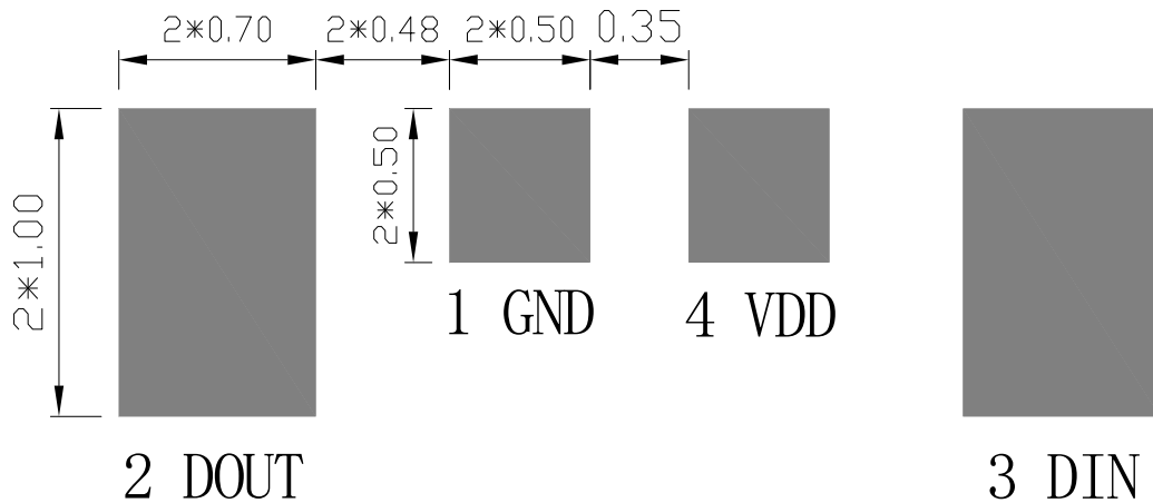
侧面贴装建议焊盘尺寸
